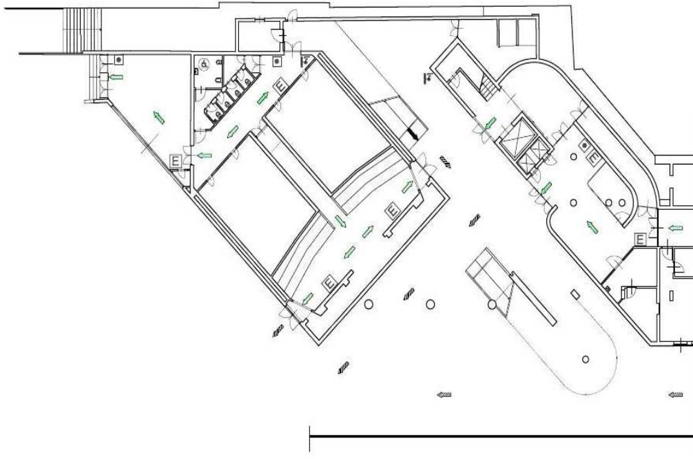
SISTEMA DI VIE DI FUGA - PIANO TERRASCALA 1:200
